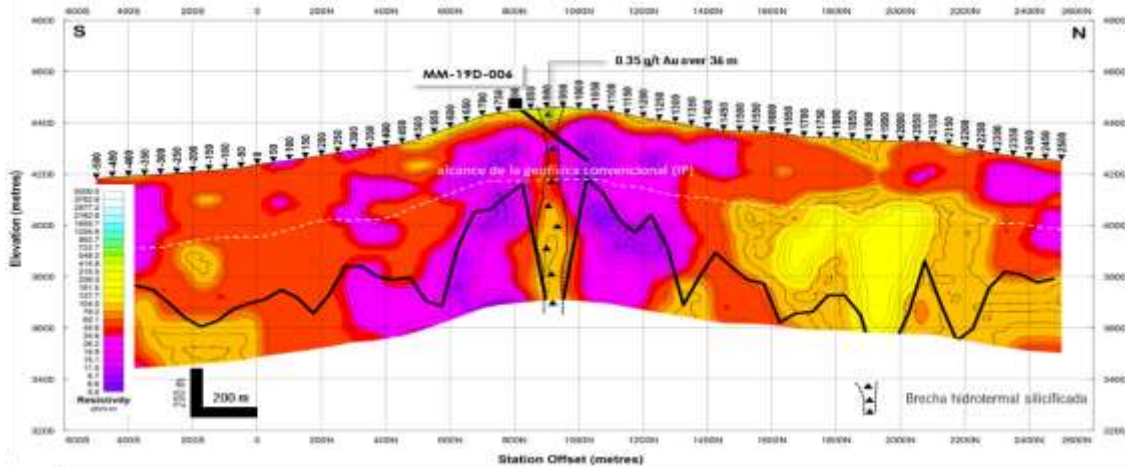
Figura 7. Sección de resistividad (CSAMT) – Línea L19800.
