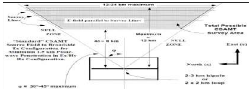
Figura 1. Configuración Estándar de un Estudio CSAMT
