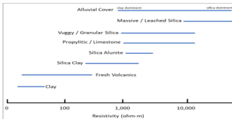
Figura 2. Rangos de resistividad de tipos de rocas.
