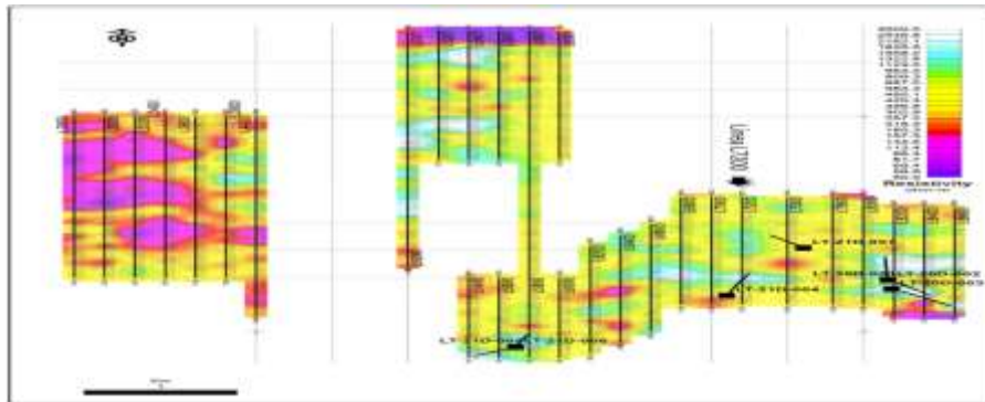
Figura 10. Estudio geofísico CSAMT en planta (-300 m).
