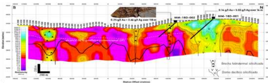
Figura 6. Sección de resistividad (CSAMT) – Línea L20800.
