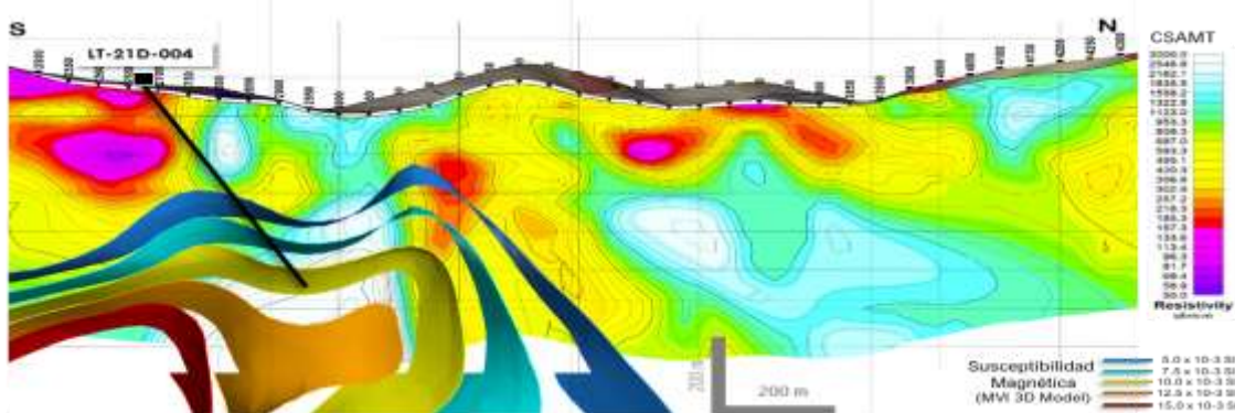
Figura 15. Sección de resistividad y susceptibilidad magnética – Línea L7200.
